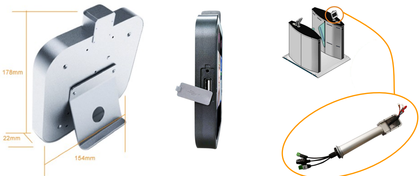
Soporte para integración en torniquetes de acceso
